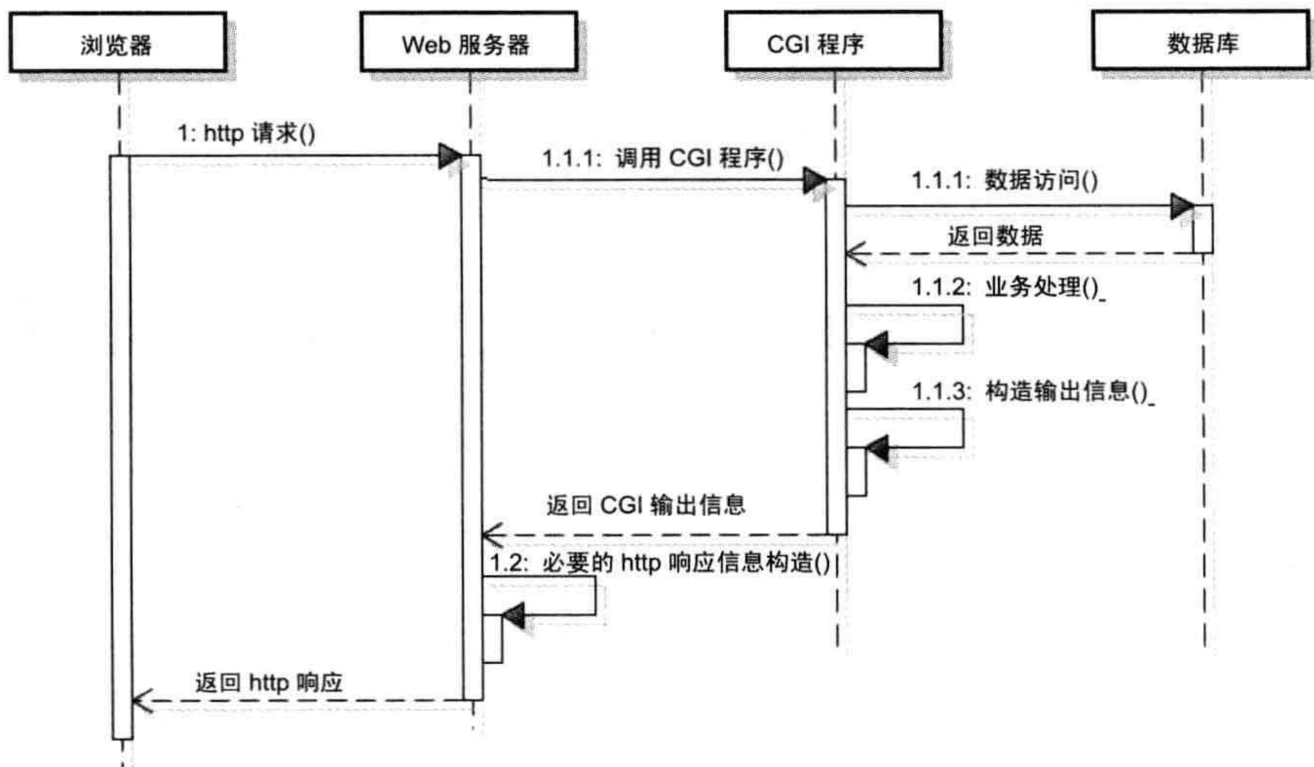
图 B.1 CGI 程序调用时序模型
