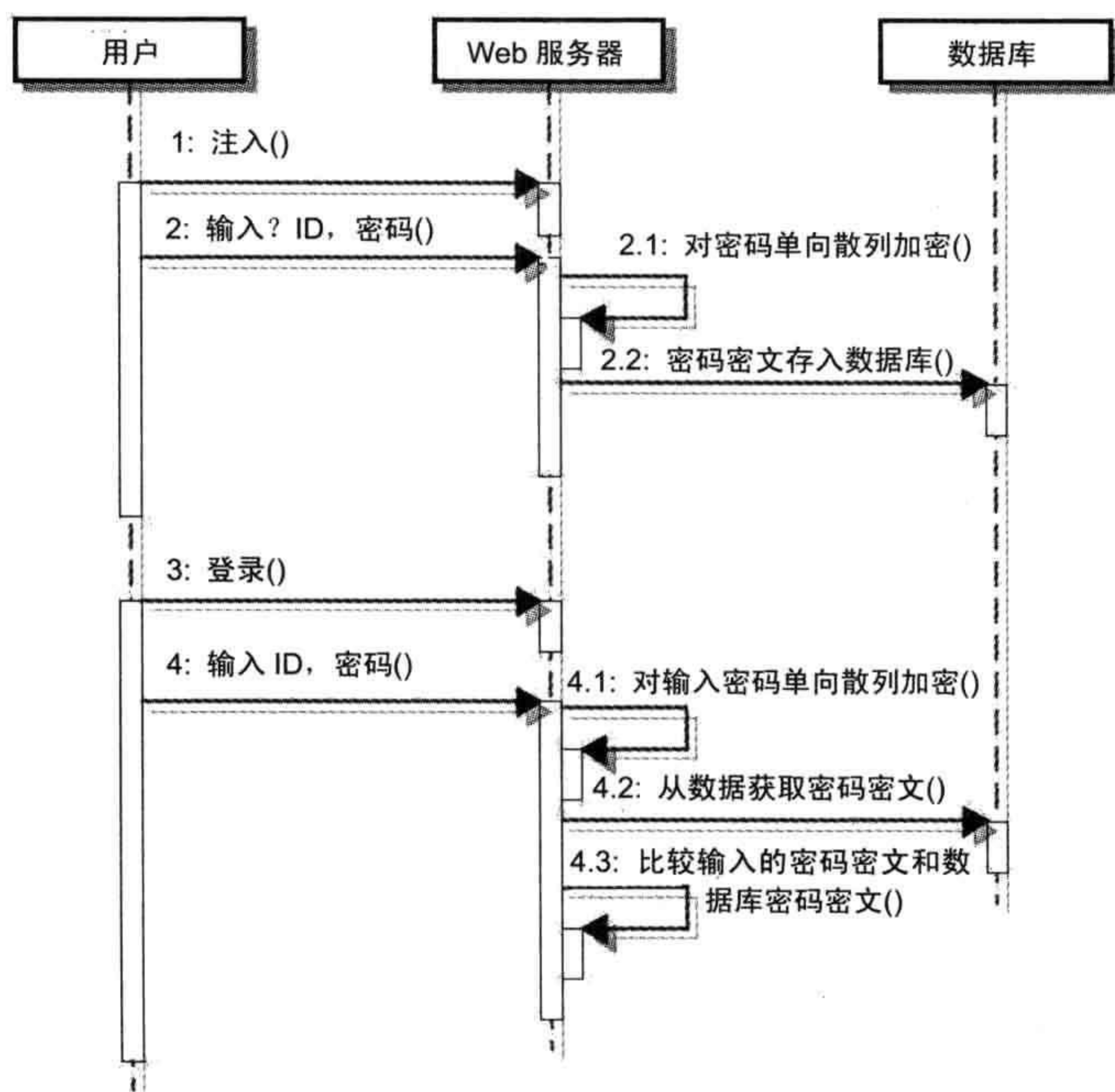
图 8.7 密码保存与验证
