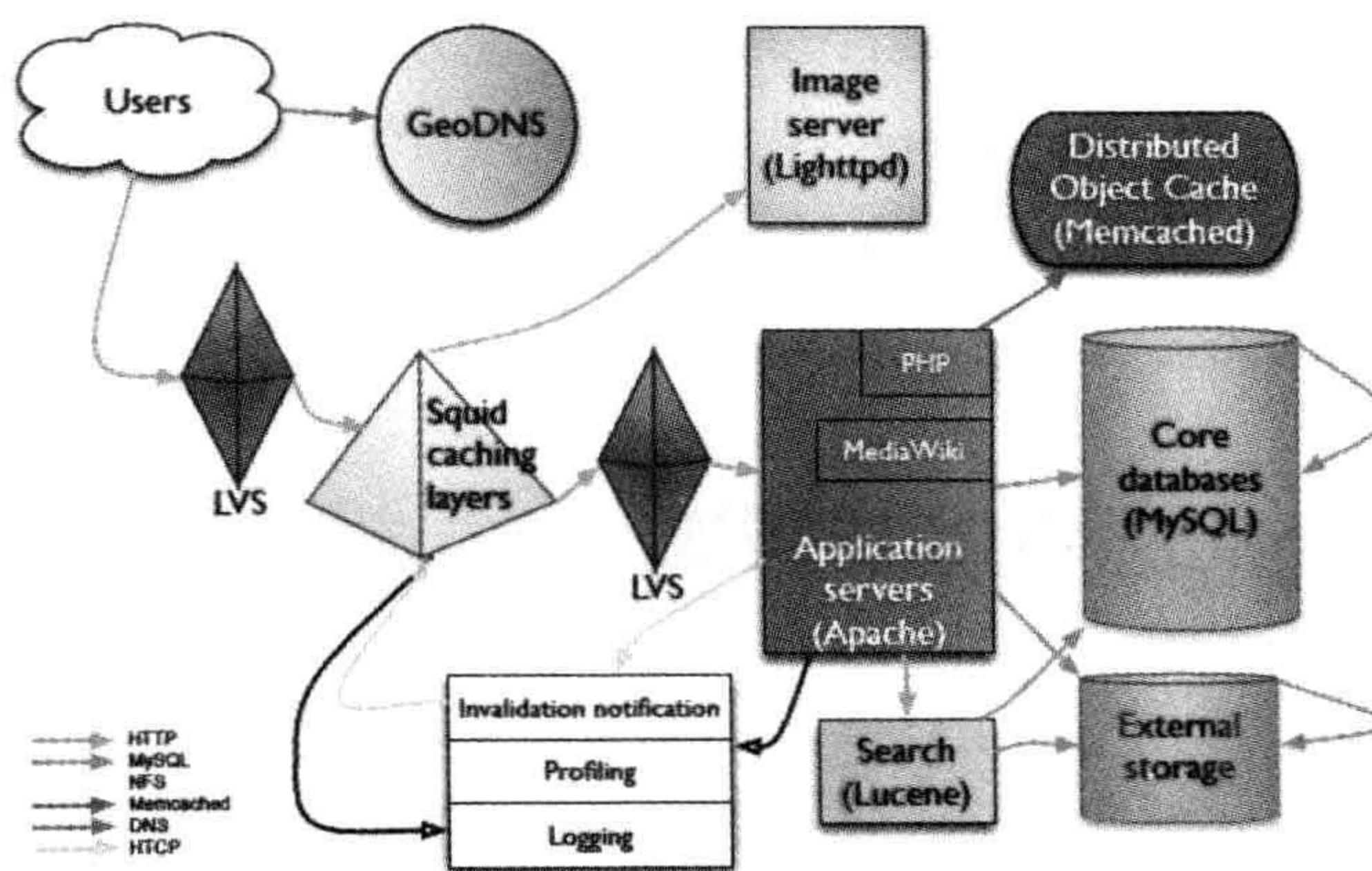
图 10.2 Wikipedia 架构图
