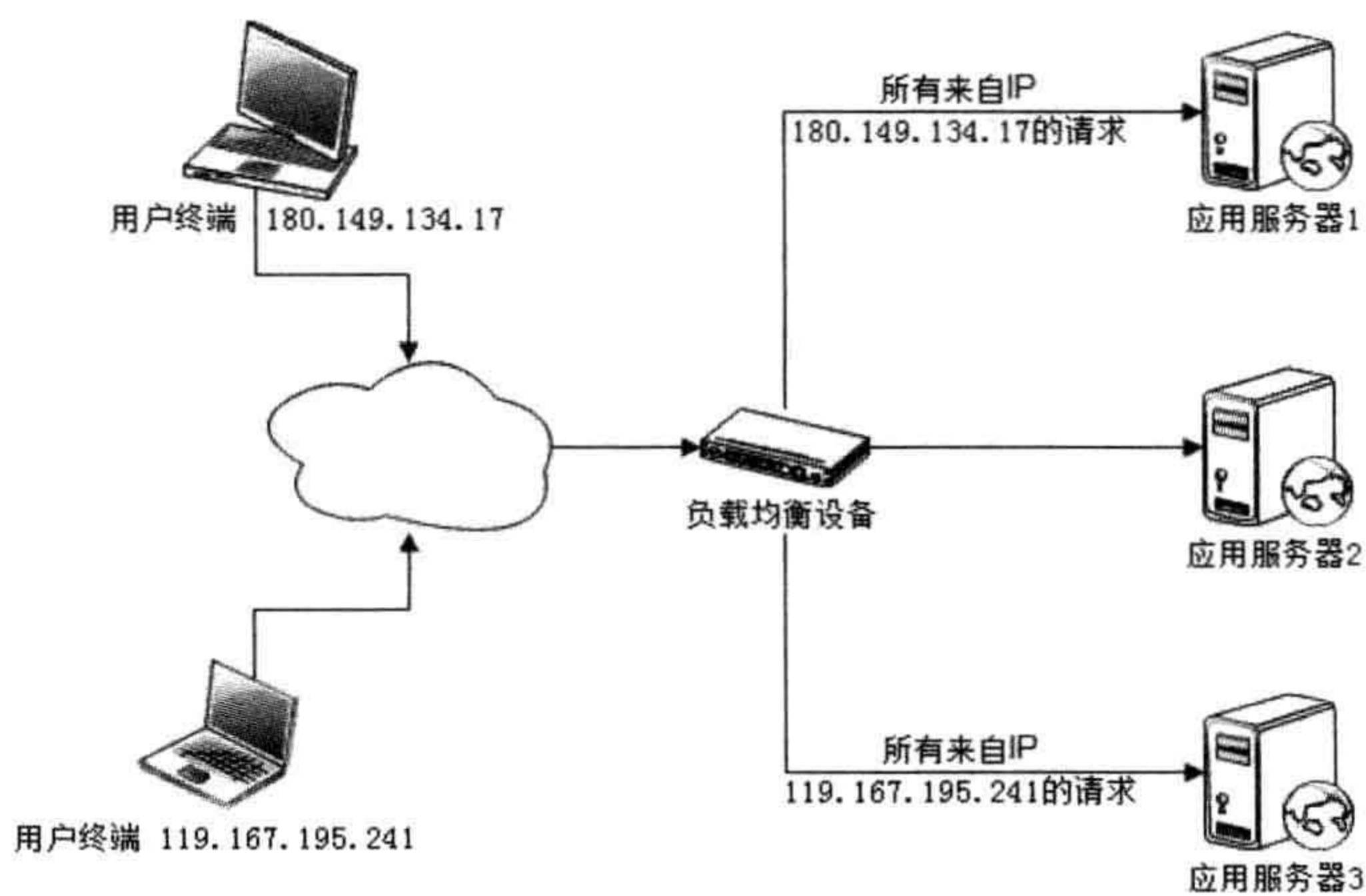
图 5.7 利用负载均衡的会话黏滞机制将请求绑定到特定服务器
