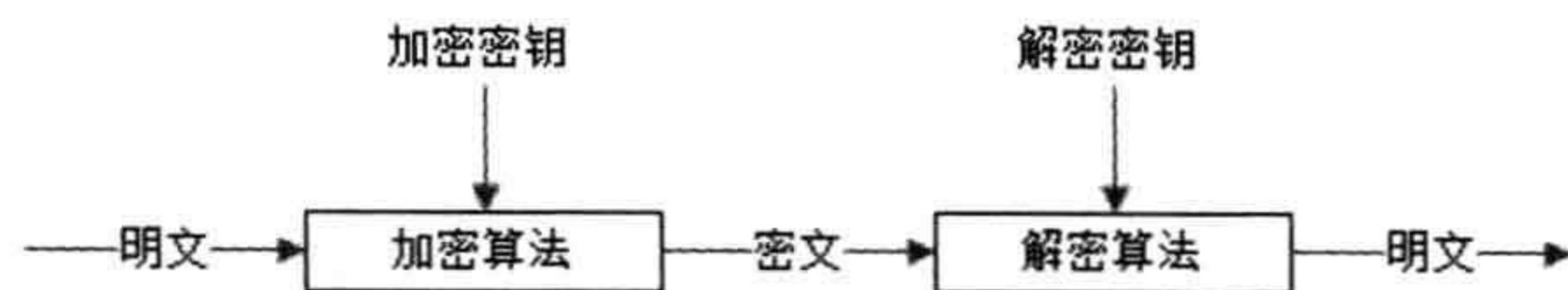
图 8.9 非对称加密
