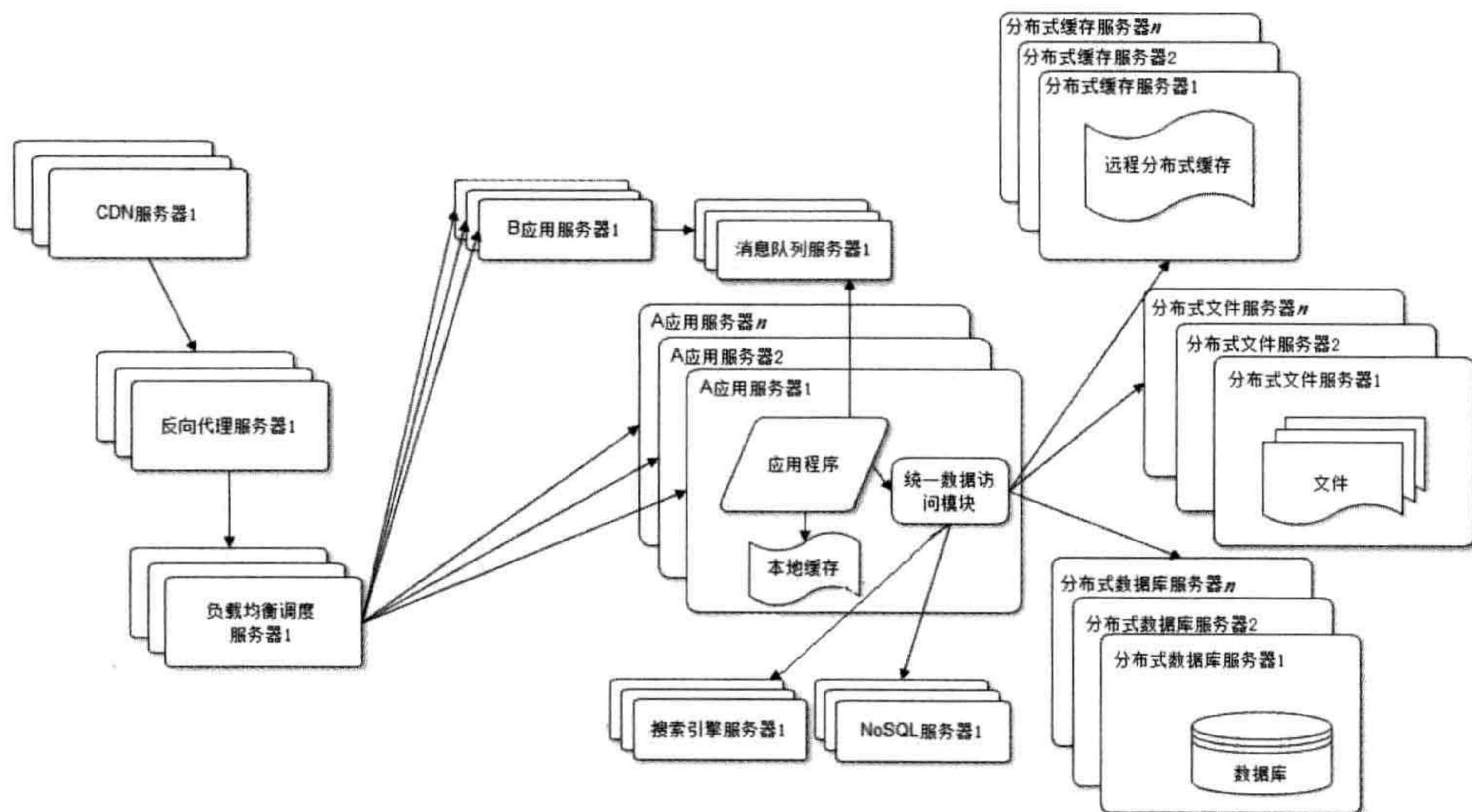
图 1.9 应用拆分
